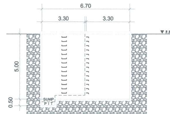
1D SECTION 3 A 3 SCALE: 1 : 200 M
