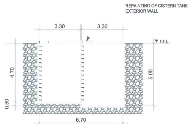
1C SECTION 2 A 3 SCALE: 1 : 200 M
