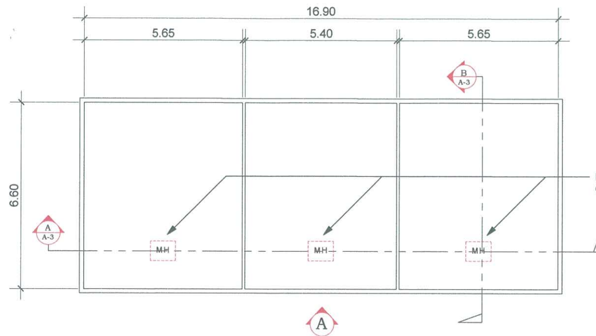
1A FLOOR PLAN SCALE: 1 : 150 M
