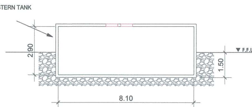
1B ELEVATION A SCALE: 1 : 150 M
